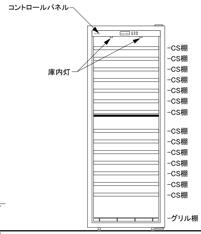
【内部正面図】
