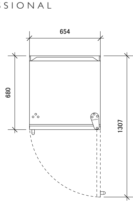
【上面図】
